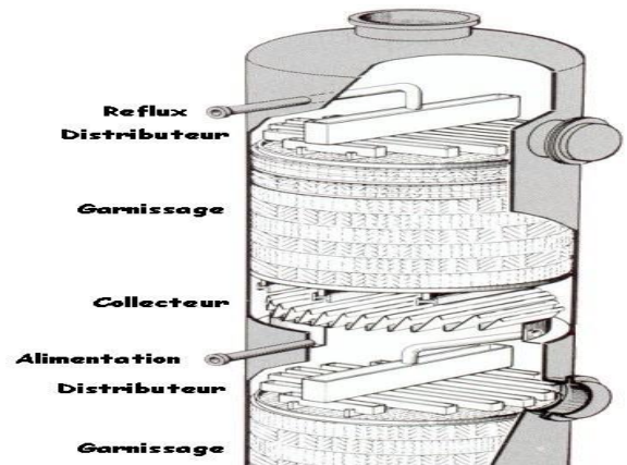
Figure VI.10. Schéma d'une colonne d'absorption a garnissage
