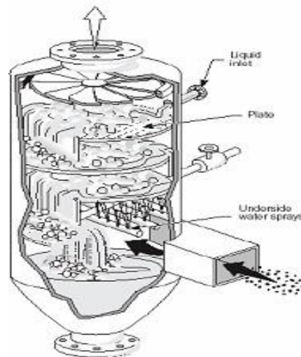
Figure VI.7. Schéma d'une colonne à plateaux à courant croisé.
