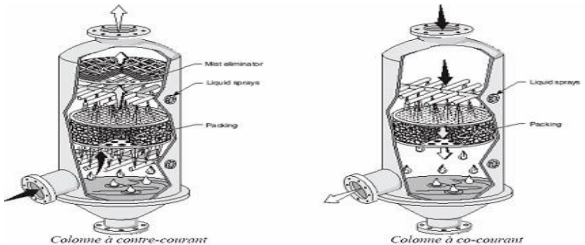
Figure VI.8. Schéma des colonnes à garnissage à contre-courant et à co-courant.
