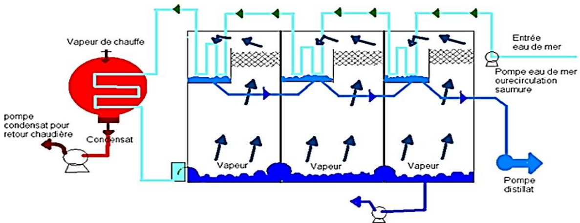
Figure III.8. Schéma Multiples du plan MSF
