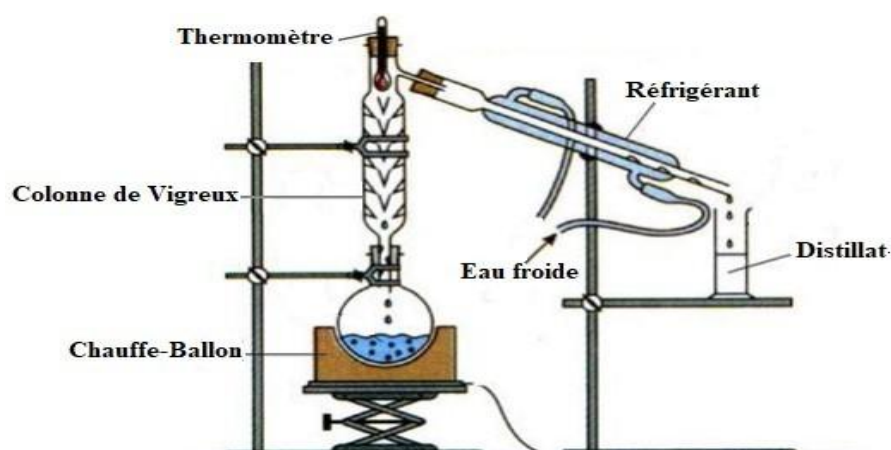
Figure III. 6. Schéma d'une distillation fractionnée
