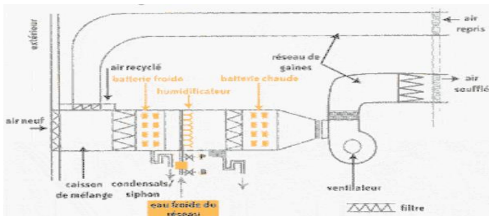
Figure I.3 : Centrale de traitement d'air.
