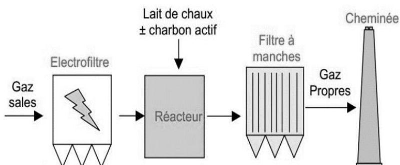
Figure II.2. Procédé semi-humide (source : de MR Julien Bertholon).
