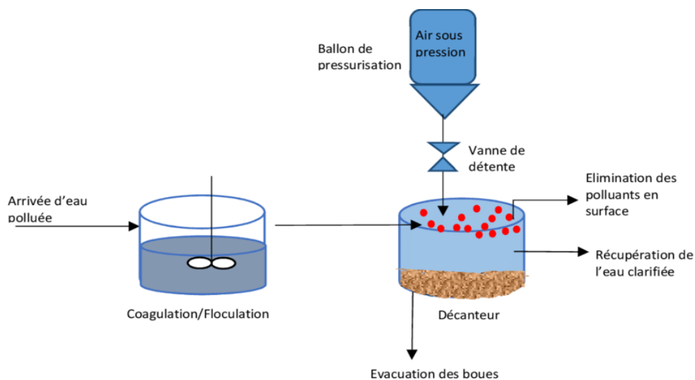
Figure III. 3 : le principe du processus de flottation par air.
