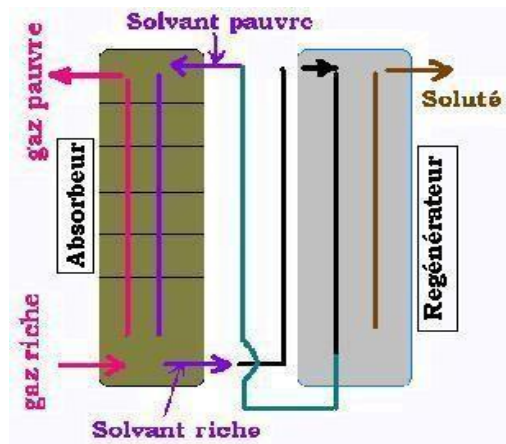
Figure IV.3. Schéma d'une colonne d'absorption avec régénération de solvant.
